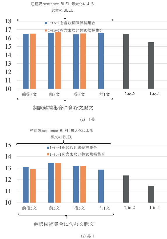
図 4 逆翻訳 sentence-BLEU 最大化による訳文・2-to-2 翻訳 (1 文前を文脈文とする)・1-to-1 翻訳の BLEU
