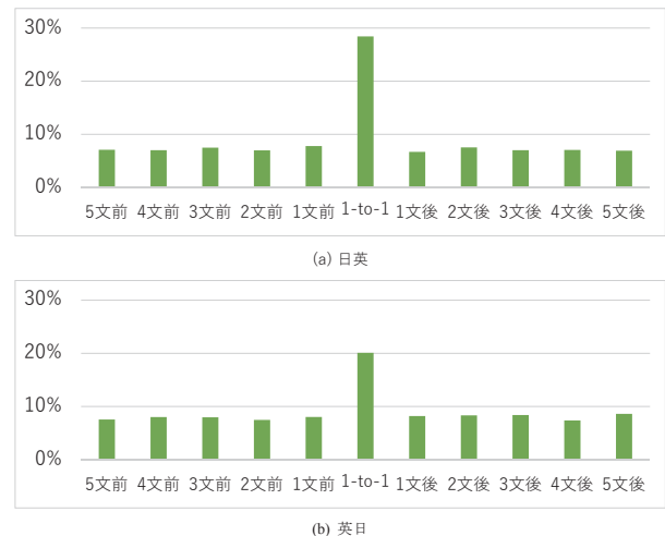
図 6 逆翻訳 sentence-BLEU 最大位置の分布
