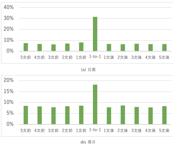
図 5 強制逆翻訳確率最大位置の分布
