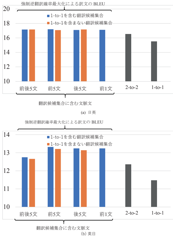
図 3 強制逆翻訳確率最大化による訳文・2-to-2 翻訳 (1 文前を文脈文とする)・1-to-1 翻訳の BLEU
