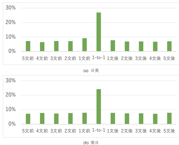
図1 オラクル翻訳における最適文脈文位置の分布
