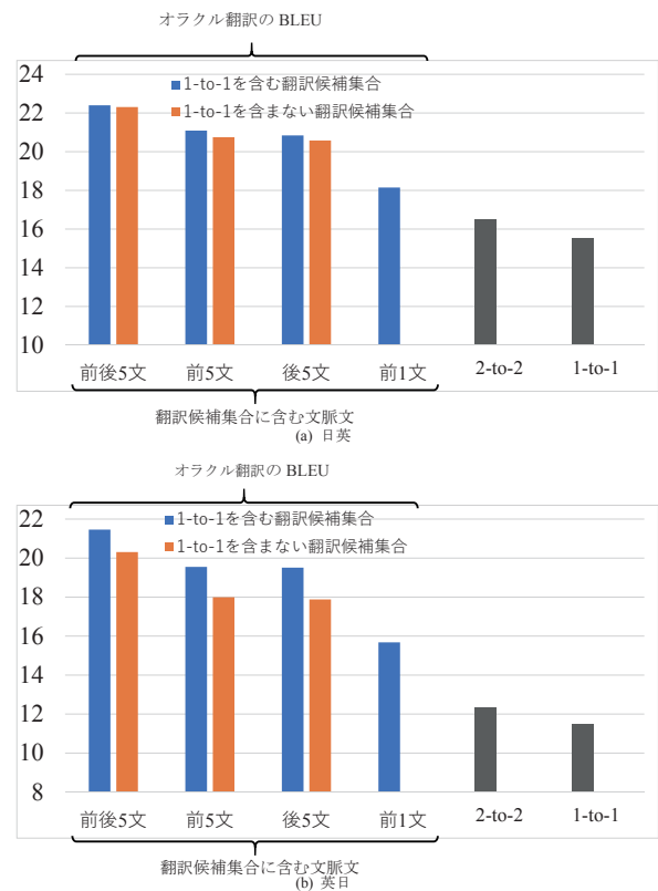
図2 オラクル翻訳・2-to-2 翻訳 (1 文前を文脈文とする)・1-to-1 翻訳の BLEU
